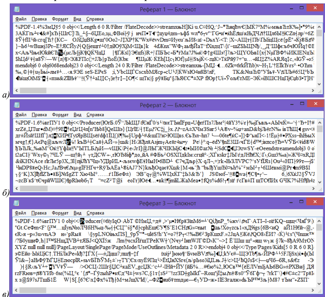
Рисунок 7. Структура исходного и зашифрованных PDF-файлов
