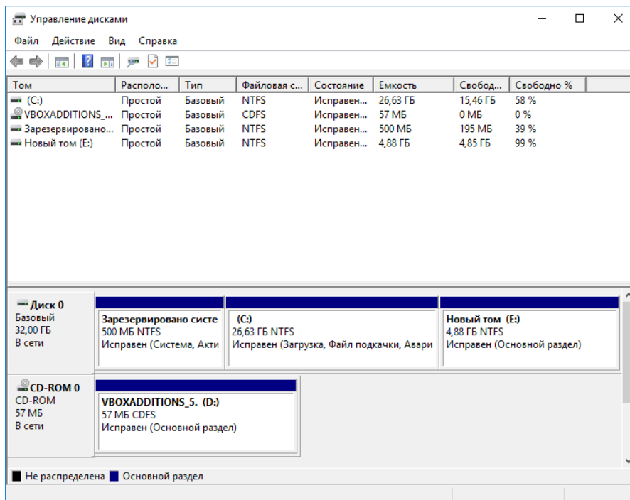
Рисунок 3.8. Новый том.
