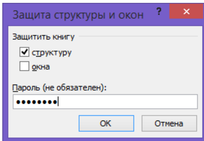
Рисунок 2.2. Защита структуры
