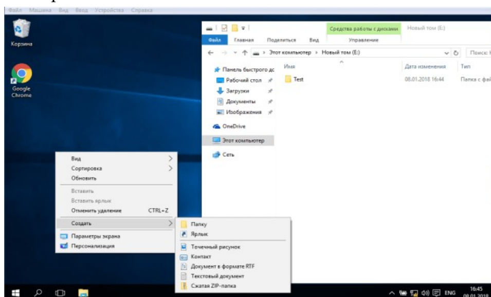
Рисунок 4.2. Создание ярлыка .
