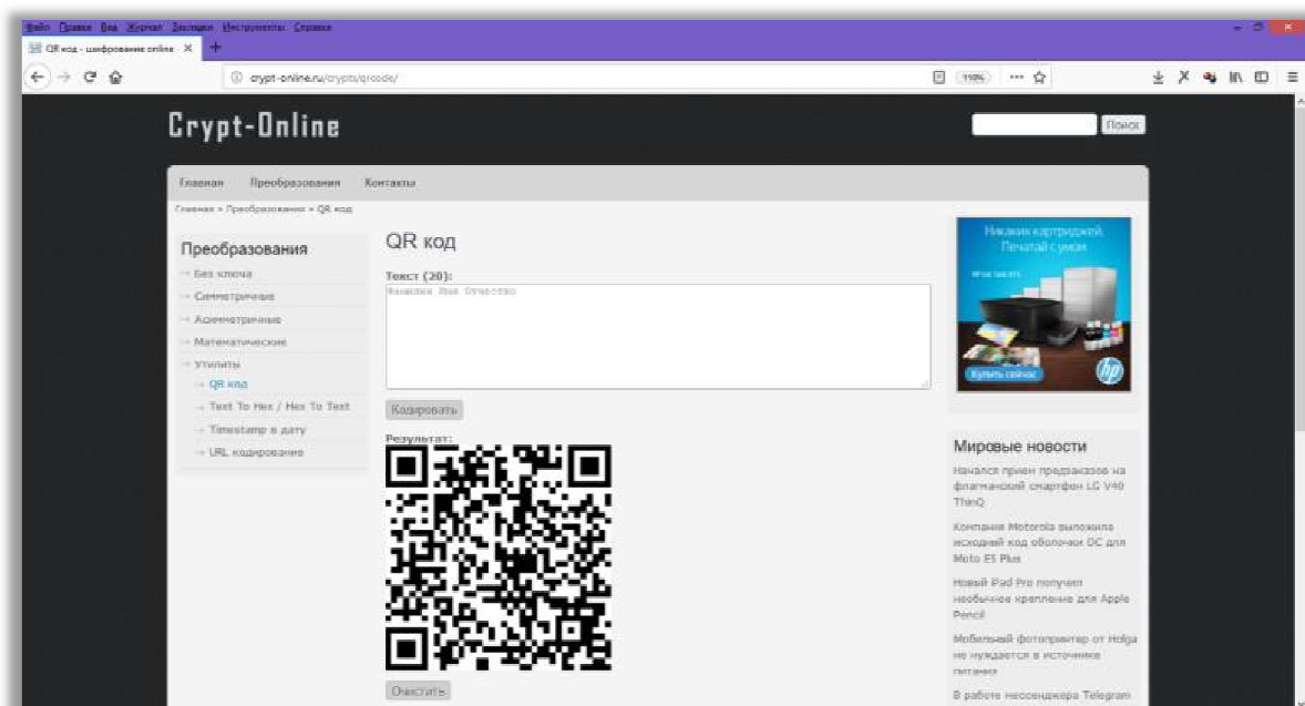
Рисунок 1.1. Создание QR-кодов.
